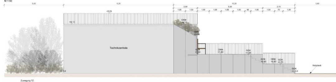
Ansicht C-C' M 1:50
