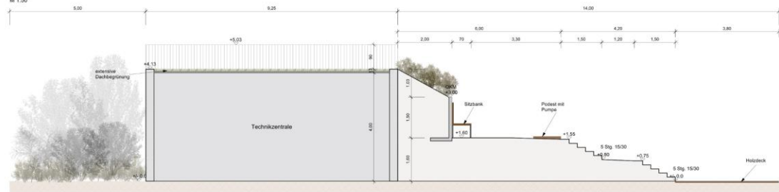
Schnitt B-B' M 1:50
