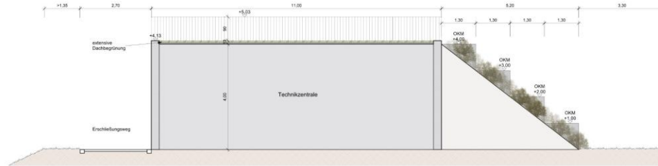
Schnitt B-B' M 1:50
